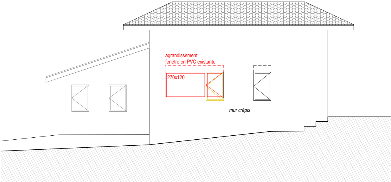
0. Façade Nord
