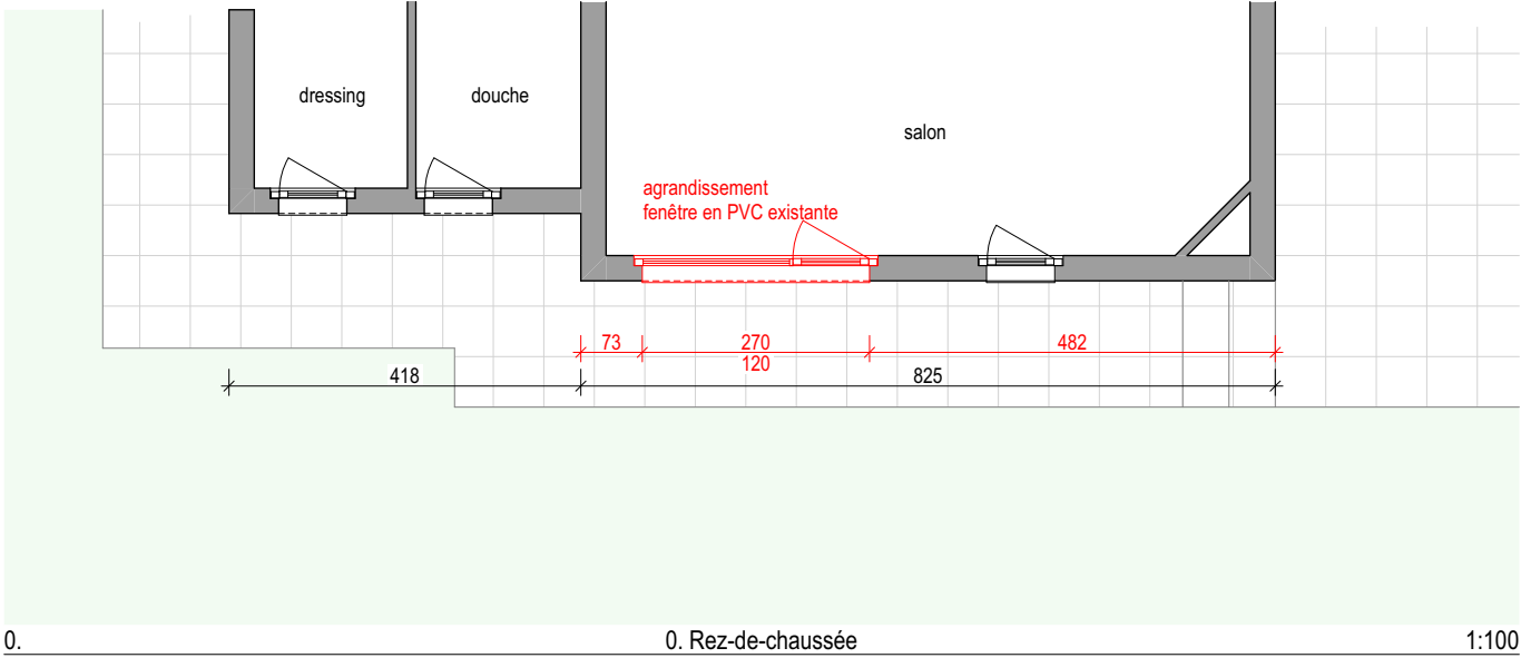
0. 0. Rez-de-chaussée 1:100
